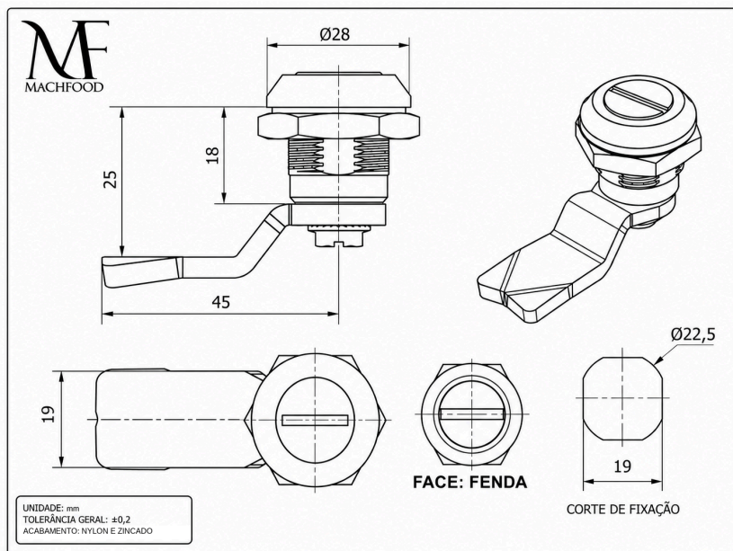
DESENHO DIMENSIONAL (mm) · VISTAS, CONJUNTO E CORTE DE FIXAÇÃO
